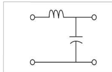
滤波电路
