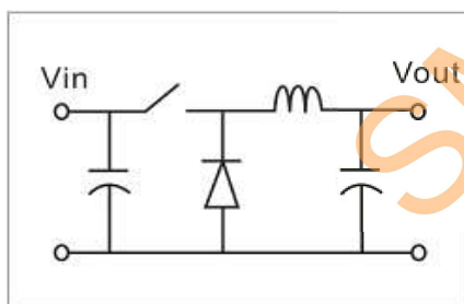
输入、输出平滑电路
